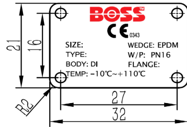
DN50-DN80
